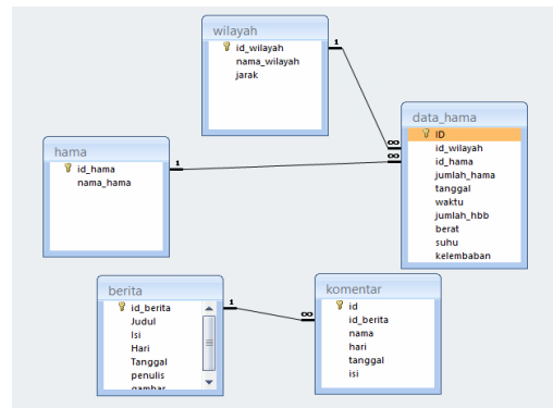
Gambar 4 ERD Sistem
