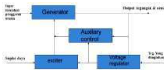
Gambar 5 Blok diagram pengontrolan sistem eksitasi.
