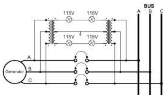
Gambar 4 indikator lampu rotasi fasa dan sama fasa
