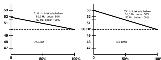
Gambar 9 Curva droop 3% dan 5%
