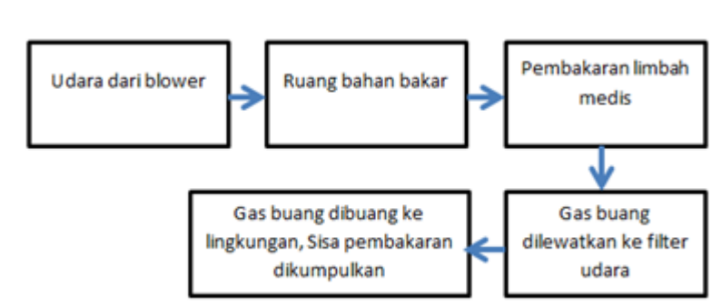
Gambar 3. Skema alat insinerator
