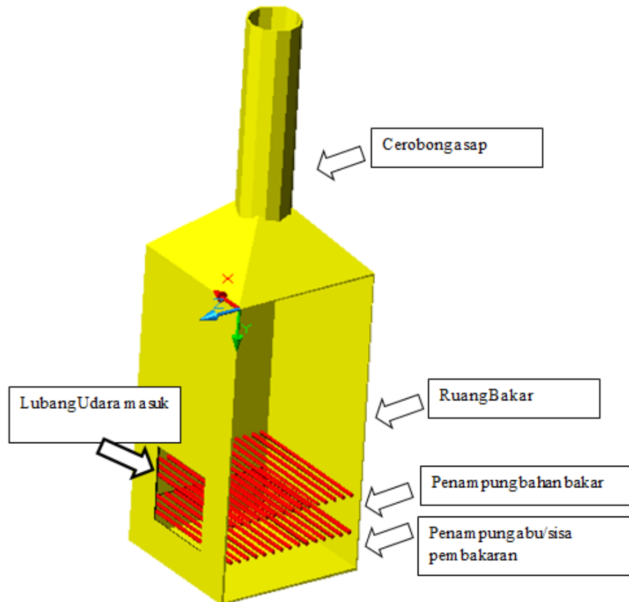
Gambar 5. Skema desain Insinerator
