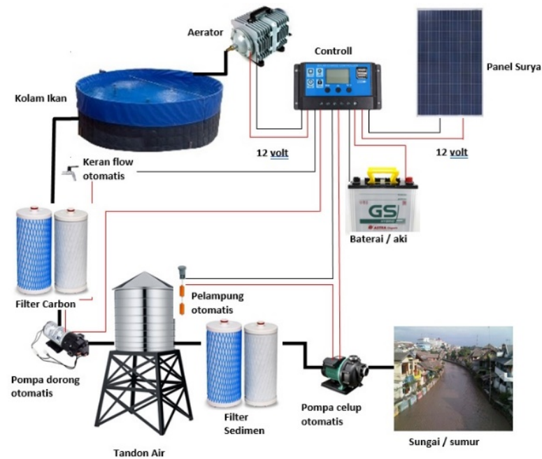
Gambar 3. Perancangan Teknologi smart tarpaulin fish
