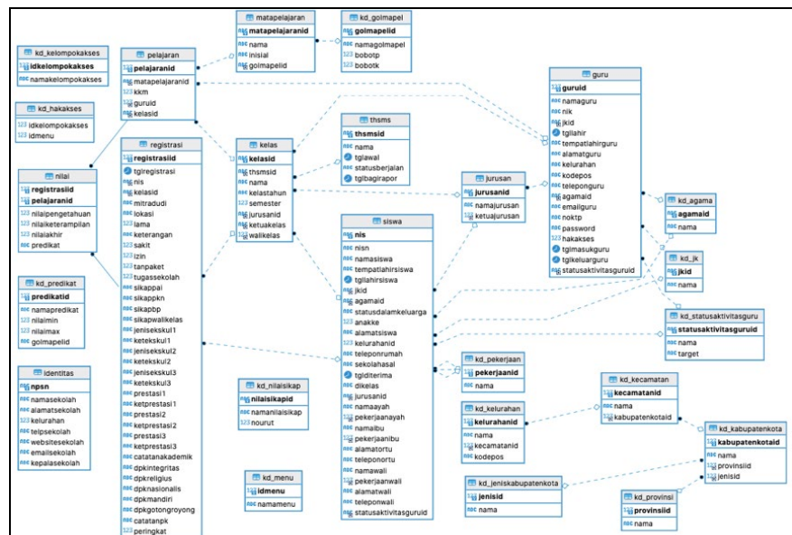
Gambar 4. Rancangan Database
