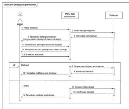
Gambar 8. Sequence Diagram Persetujuan Pemijanan
