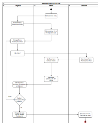
Gambar 3. Activity Diagram Peminjaman Aset
