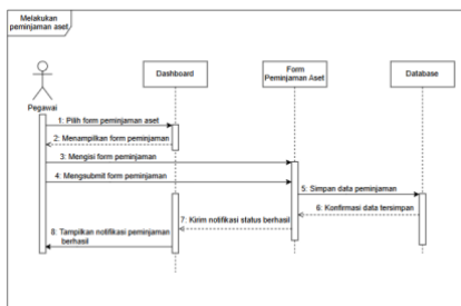
Gambar 7. Sequence Diagram Pemijanan Aset
