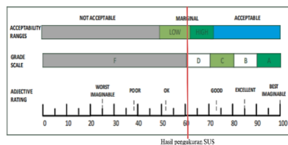
Gambar 1. Skor Hasil
