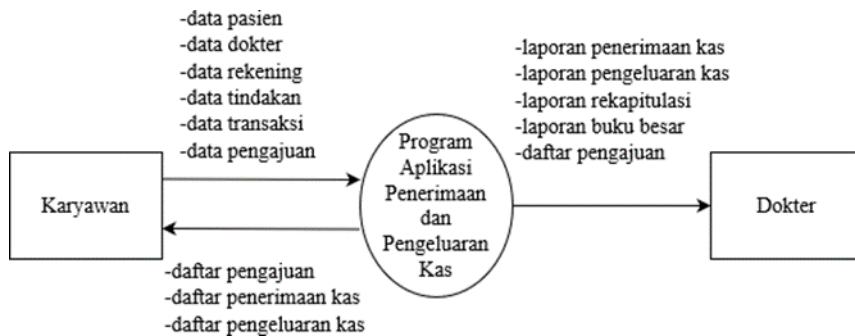
Gambar 2. Diagram Konteks
