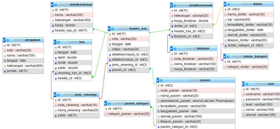
Gambar 1. Database dan Relasi Antar Tabel
