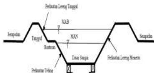
Gambar 1. Penampang Melintang Sungai (Sudaryoko, 1987).
